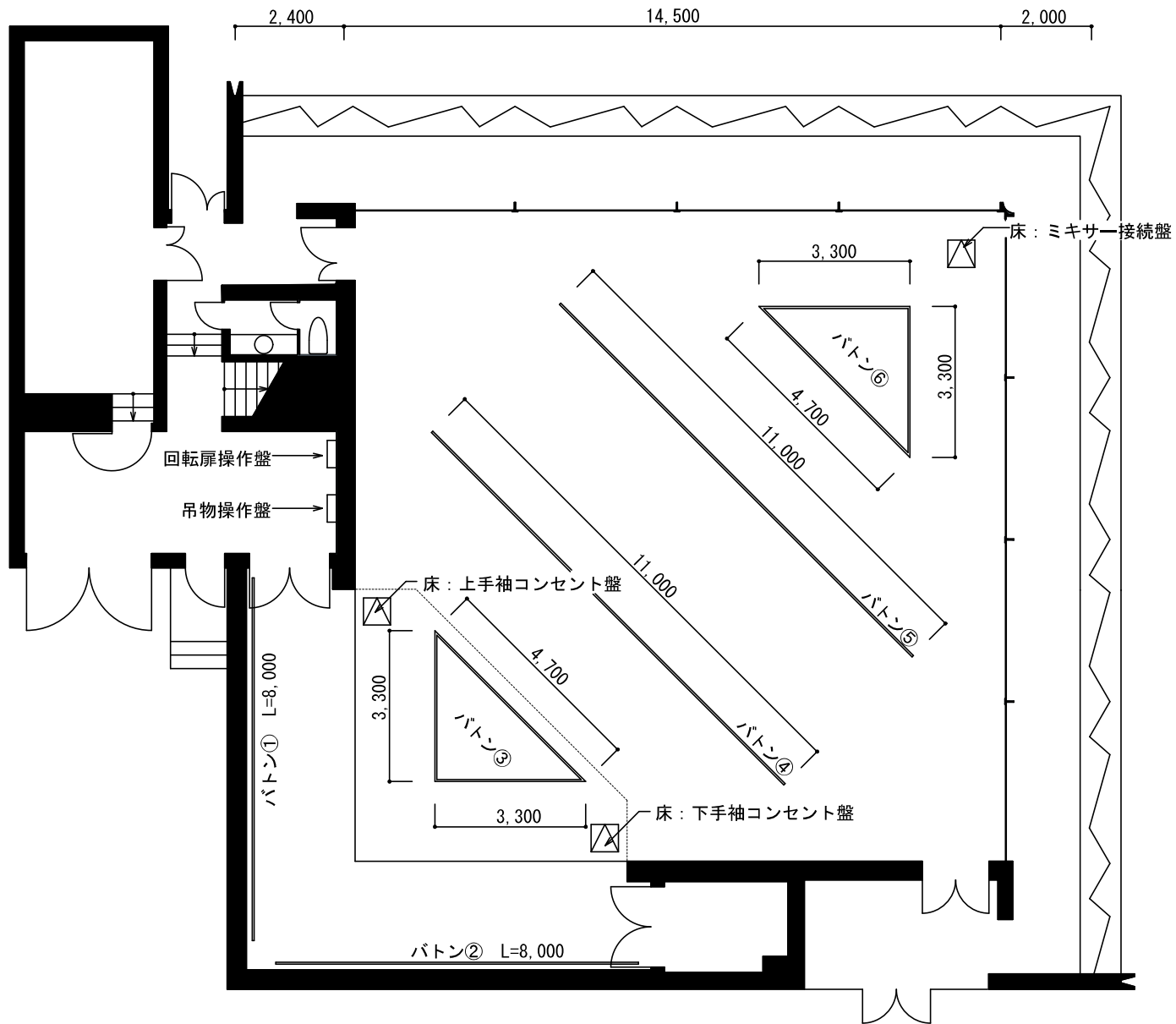
多目的ホール（キューブA） 吊物、操作・接続盤平面図
