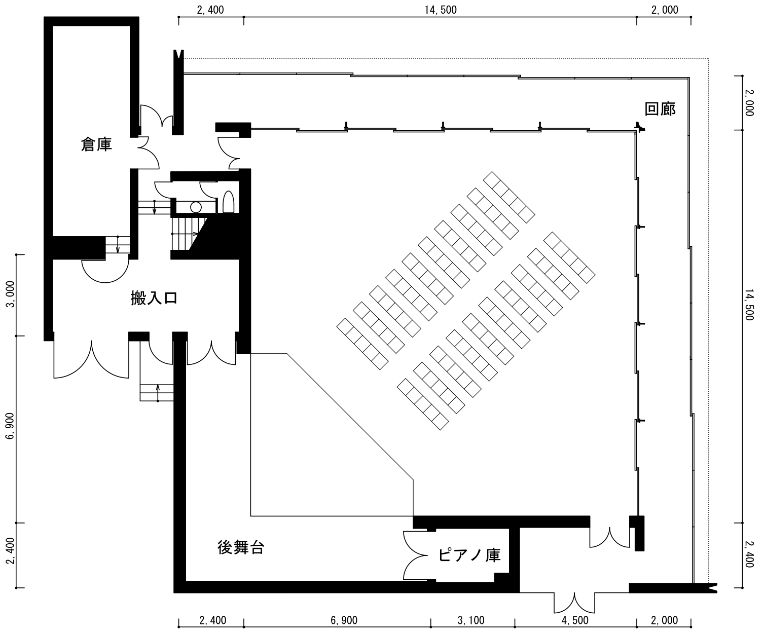
多目的ホール (キューブA)
